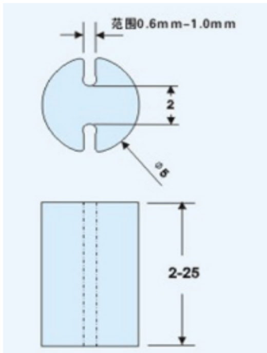
尺寸图
