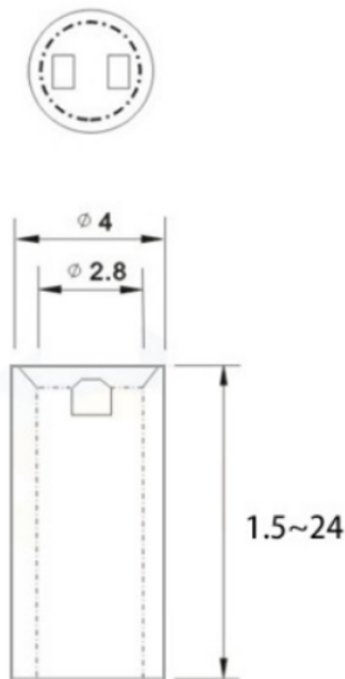
尺寸图
