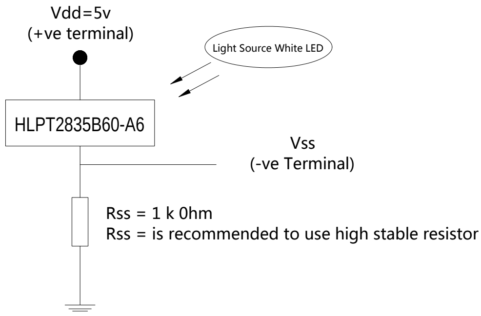
LED通用驱动电路
